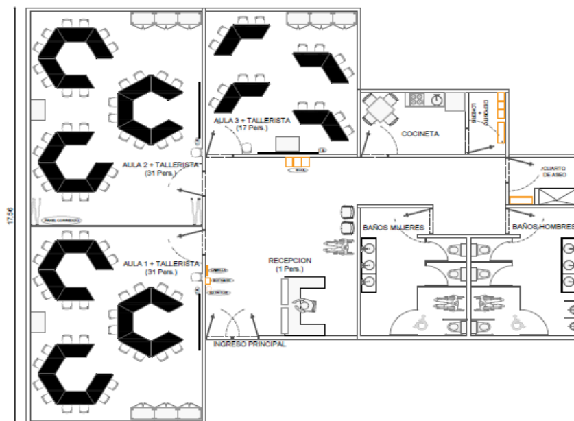
Fig. 1. Propuesta Arquitectónica Sacúdete Tipo II
