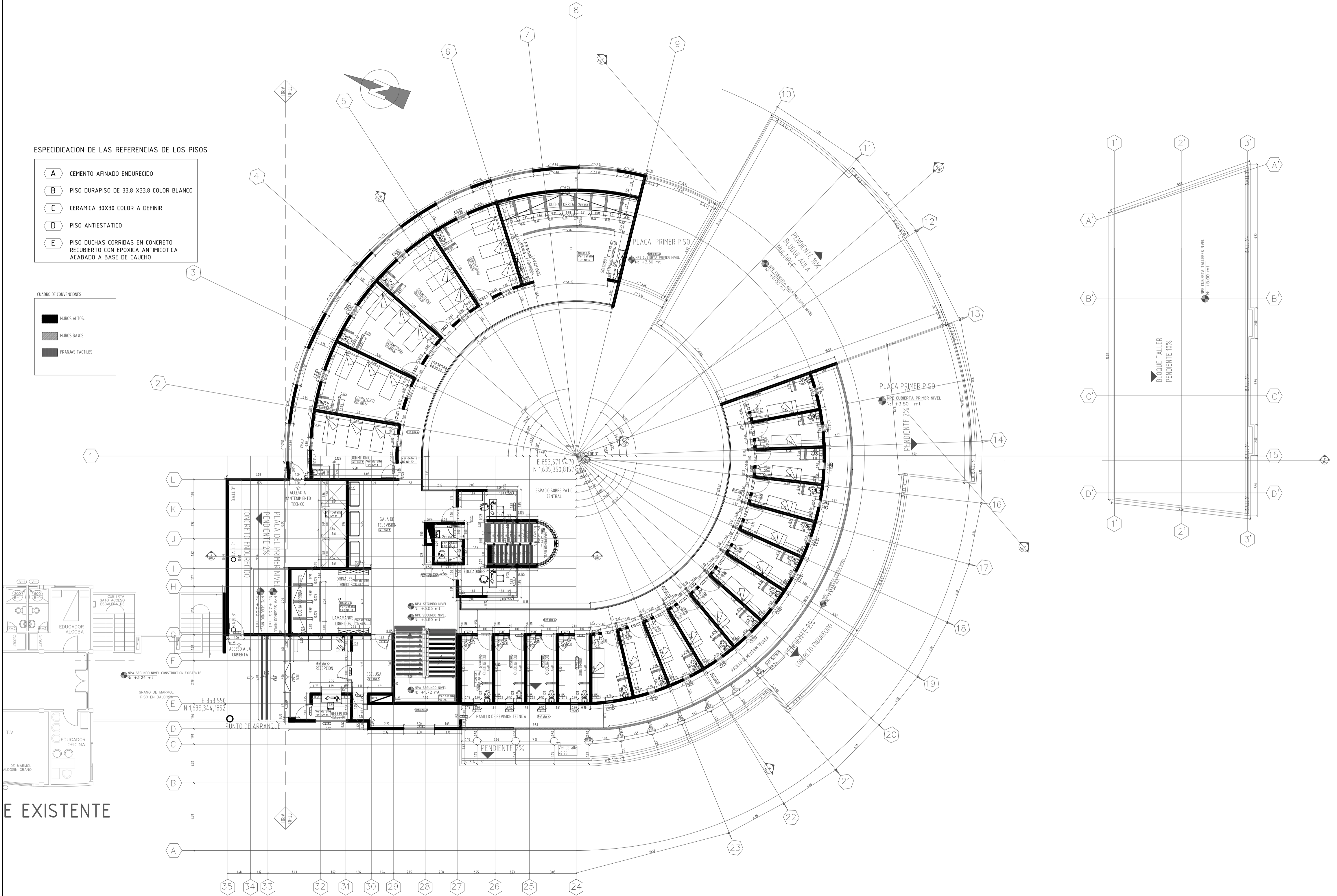
PLANTA SEGUNDO NIVEL ESCALA 1:100
