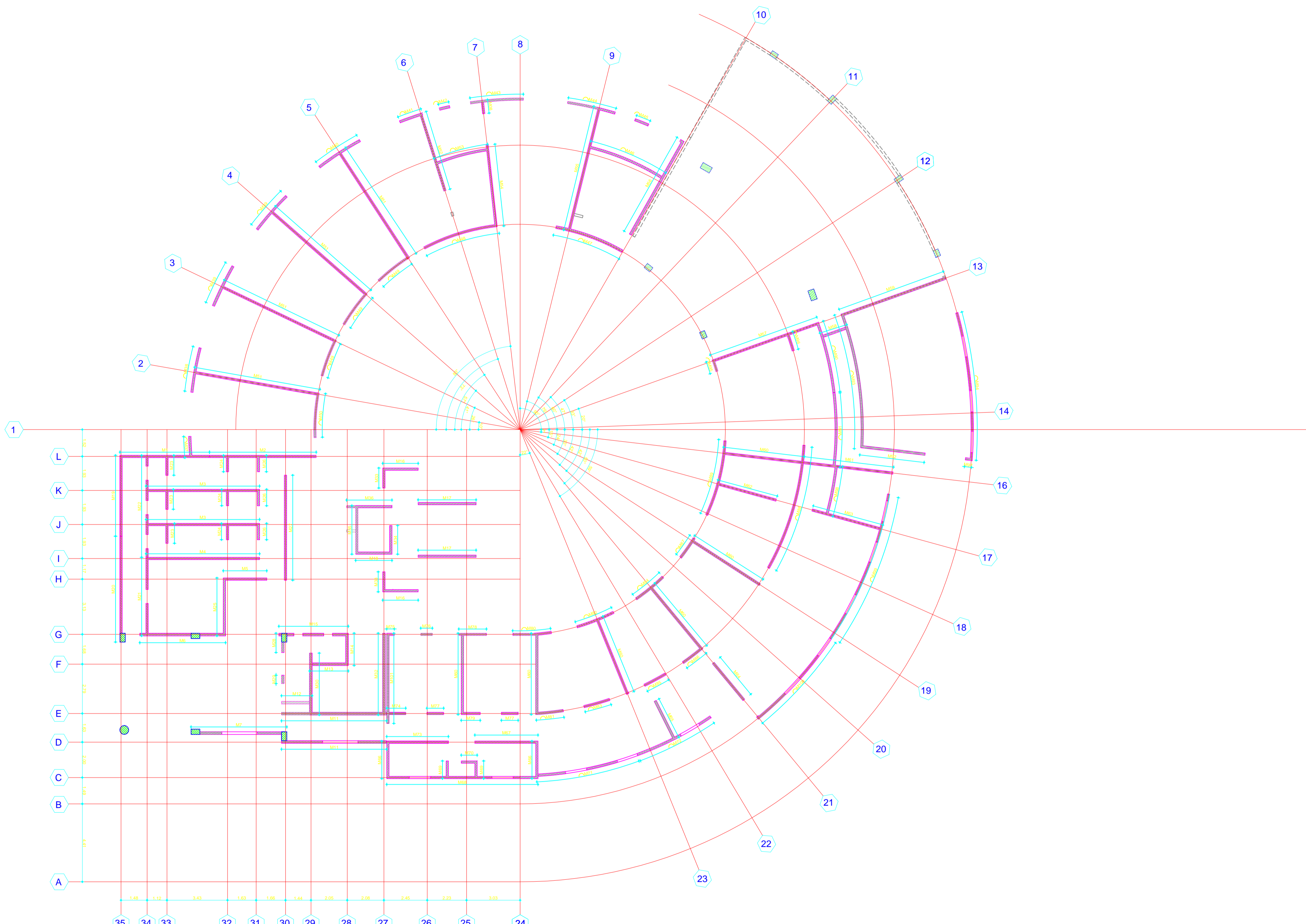
PLANTA TIPO DE MUROS PLANTA DE PRIMER PISO
