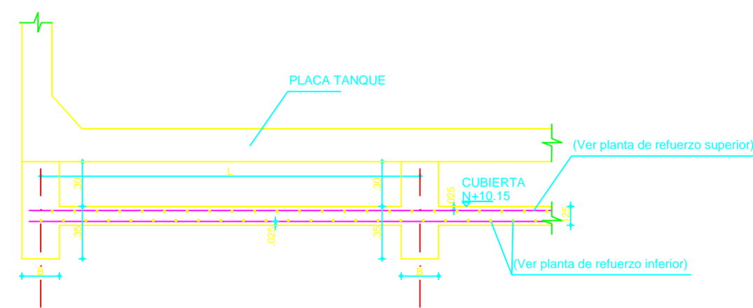
CORTE TÍPICO DE PLACA MACIZA ZONA DE TANQUE
