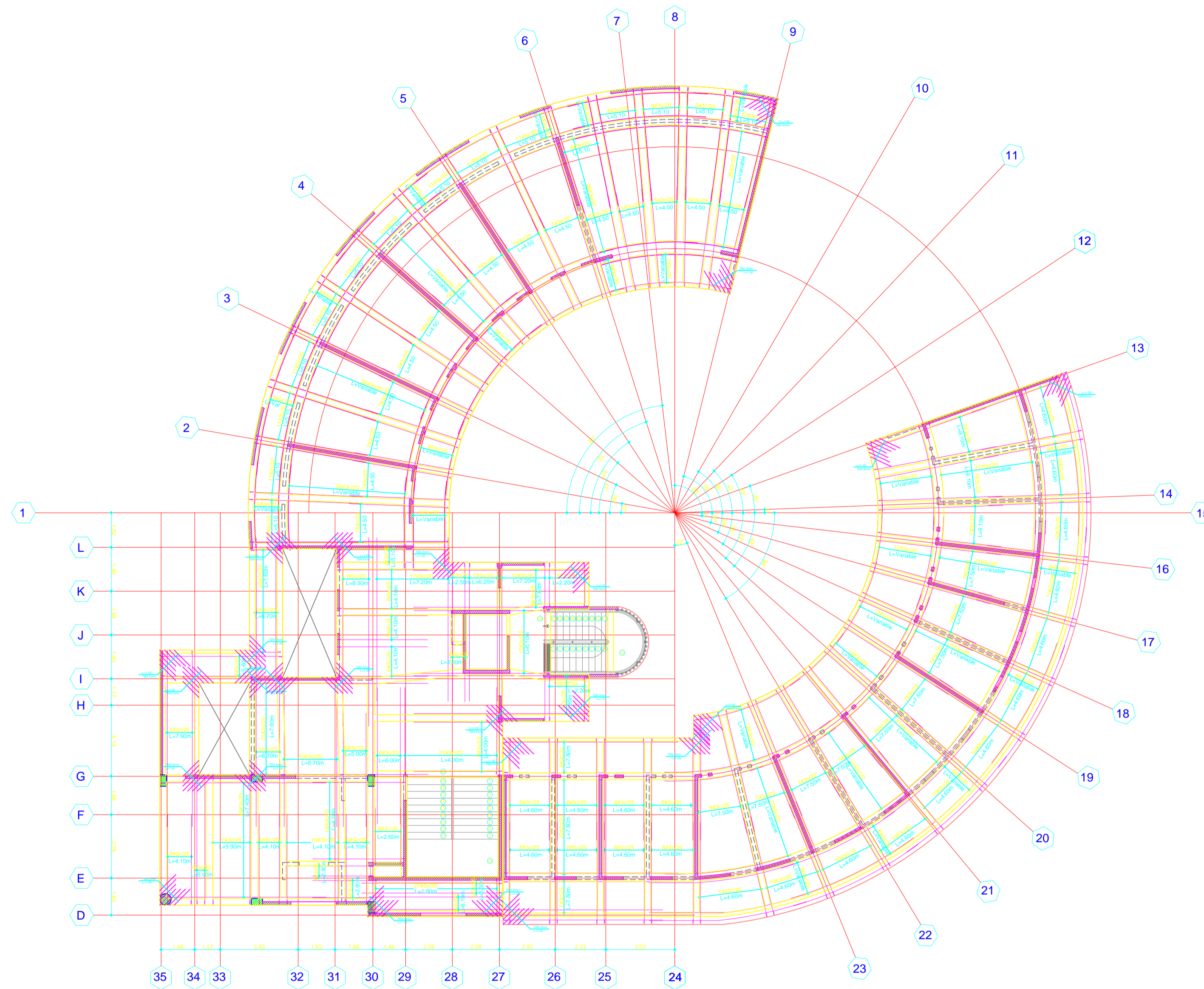
PLANTA DE REFUERZO SUPERIOR PLANTA DE TERCER PISO
