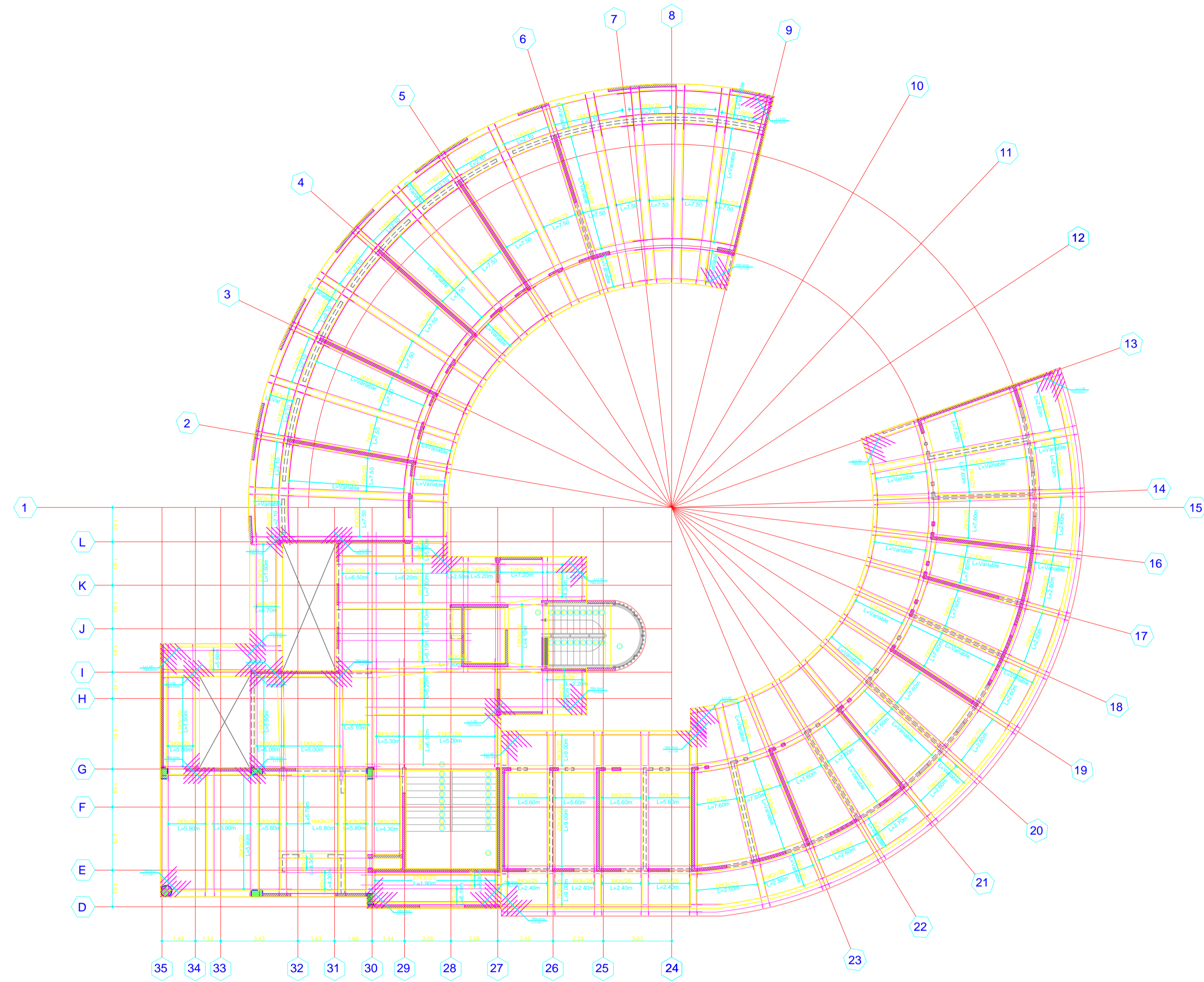
PLANTA DE REFORZO INFERIOR PLANTA DE TERCER PISO
