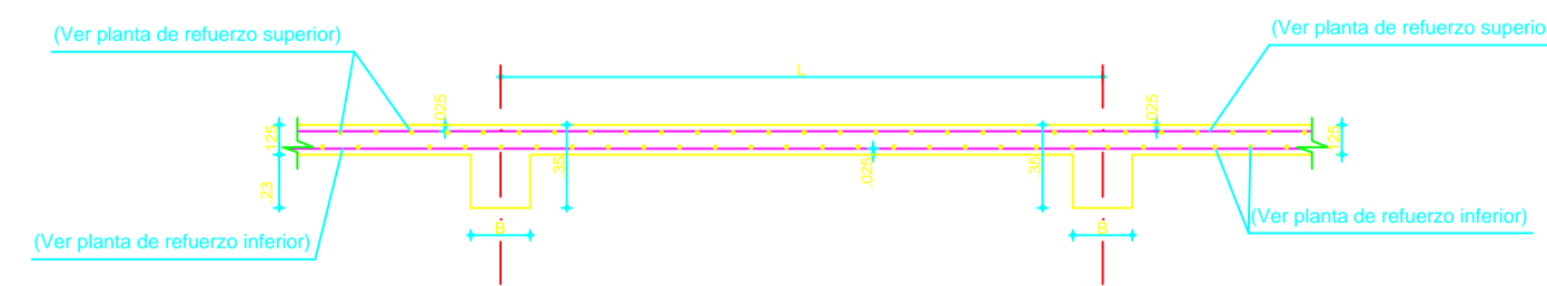
CORTE TÍPICO DE PLACA MACIZA
