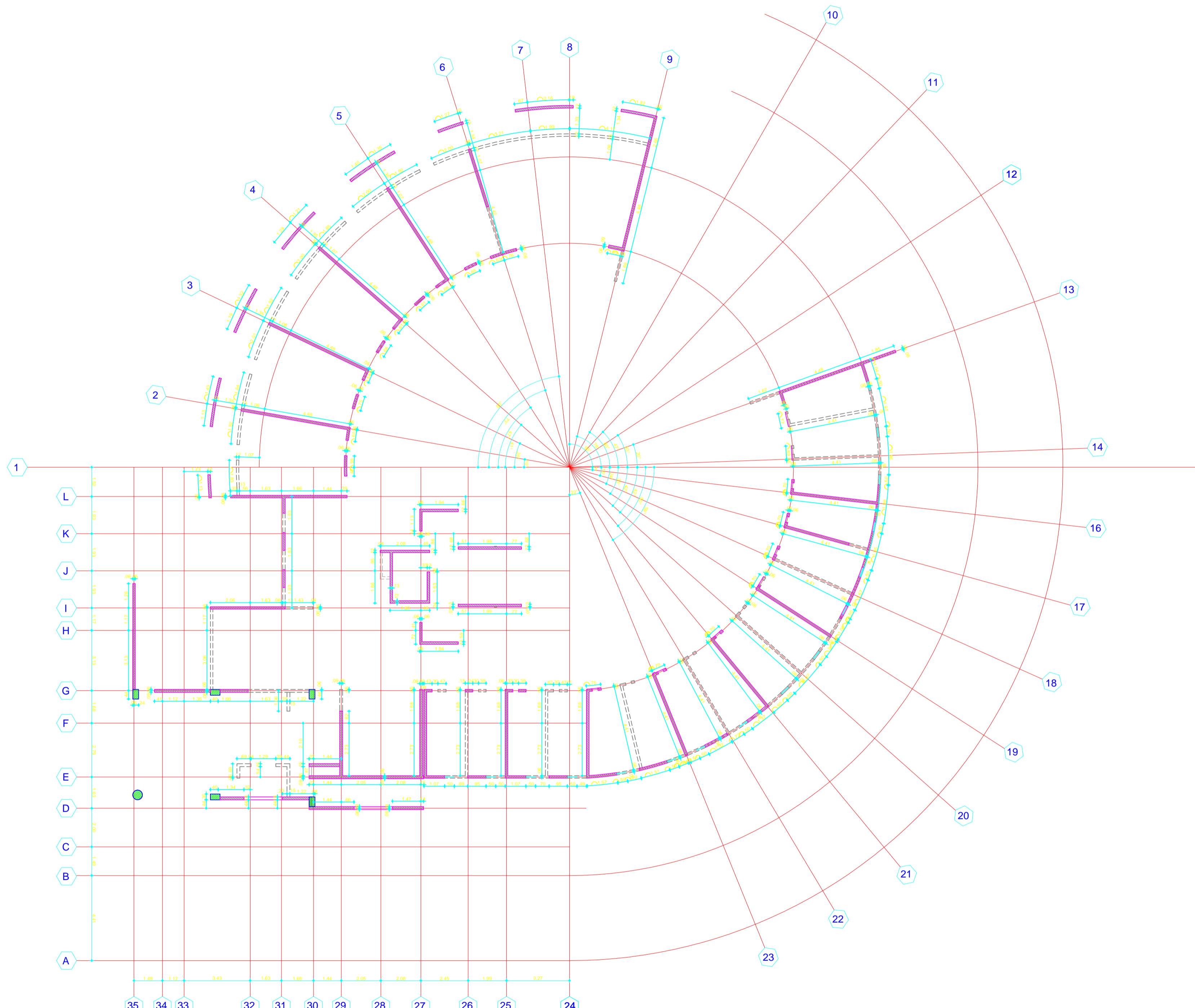
PLANTA LOCALIZACION DE MUROS SEGUNDO PISO ESCALA.....1-100
