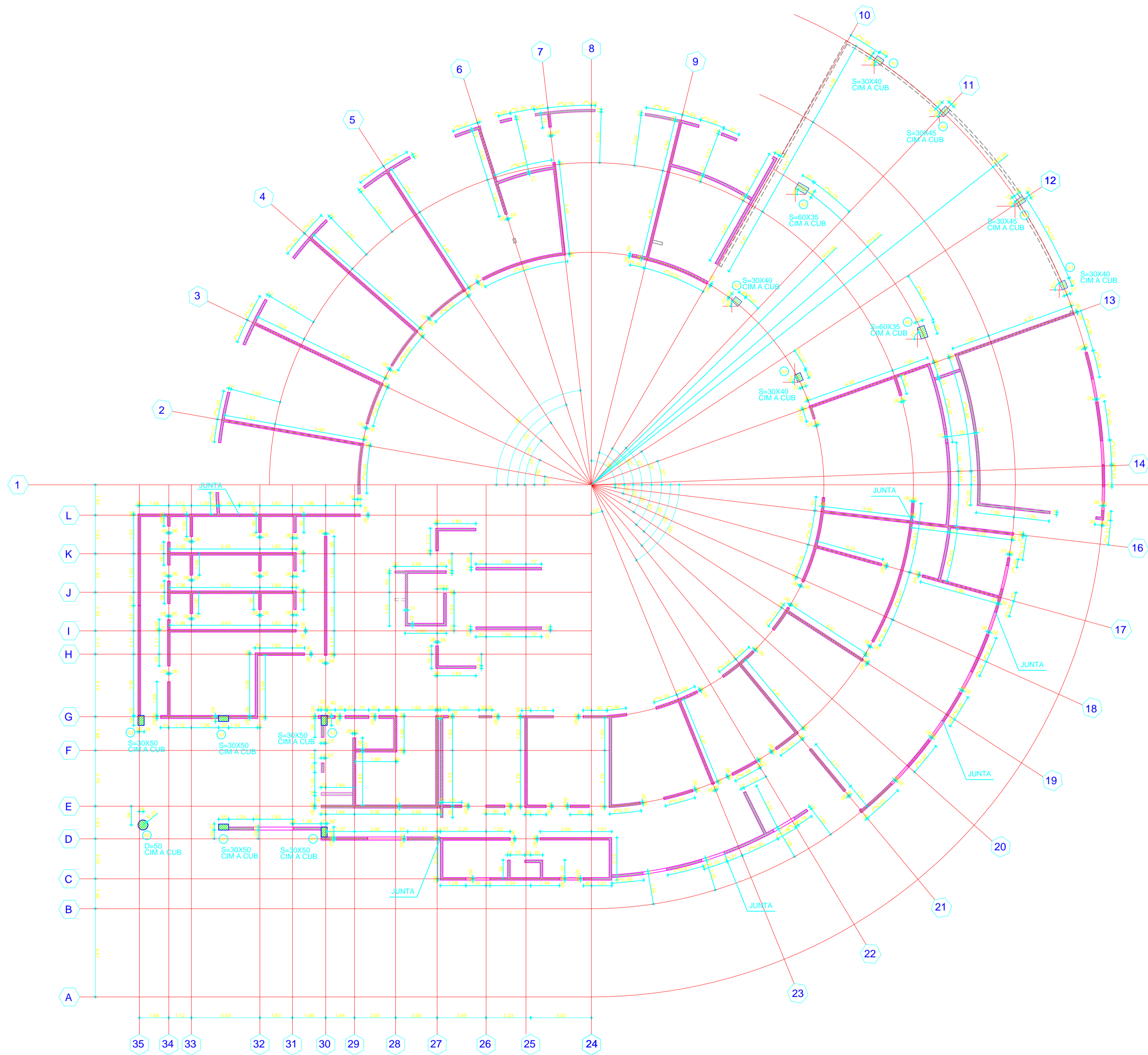
PLANTA LOCALIZACION DE MUROS PRIMER PISO
