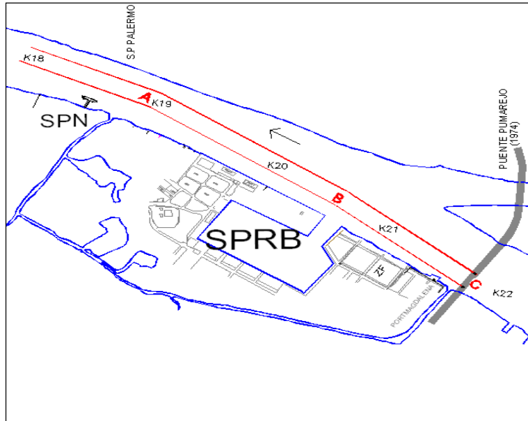
Figura 3. Ubicación del eje del canal navegable entre el K19+500 al K21+825
