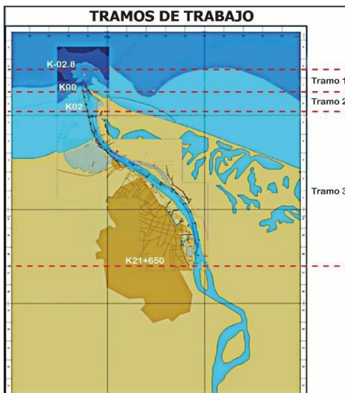
Figura 1. Tramos de Trabajo del canal navegable
