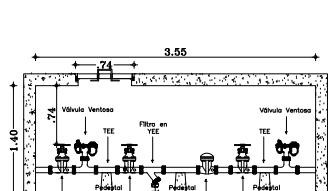
DETALLE INSTALACIÓN MACROMEDIDOR PERFIL 2. 1/2"
