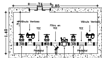
DETALLE INSTALACIÓN VÁLVULA REDUCTORA DE PRESIÓN PERFIL 2. 1/2"
