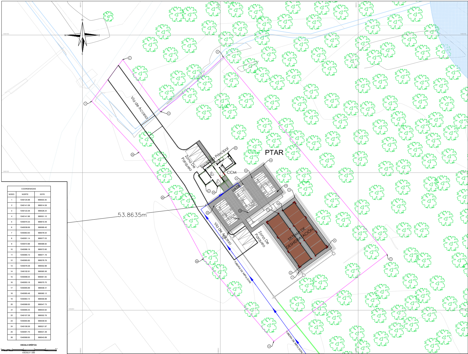
LOCALIZACIÓN DE ESTRUCTURAS DE LA PTAR
