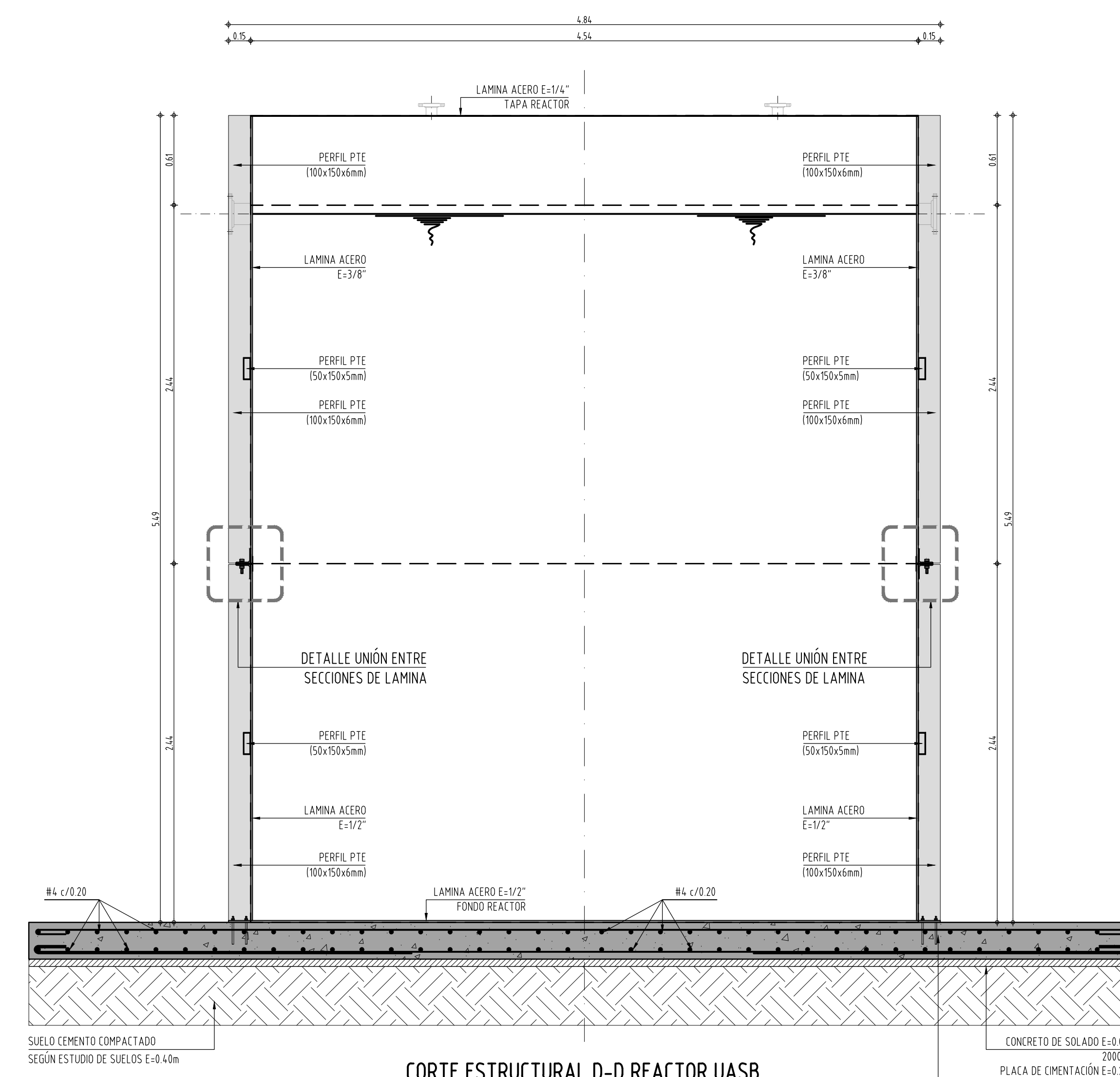
CORTE ESTRUCTURAL D-D REACTOR UASB
