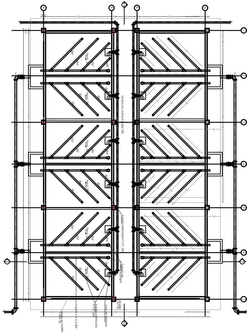
PLANTA DE PRIMER PISO 1:50
