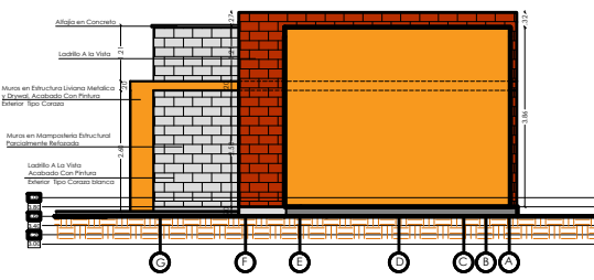
FACHADA LATERAL DERECHA 1:50
