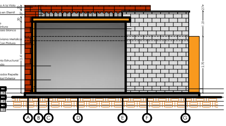
FACHADA LATERAL IZQUIERDA 1:50
