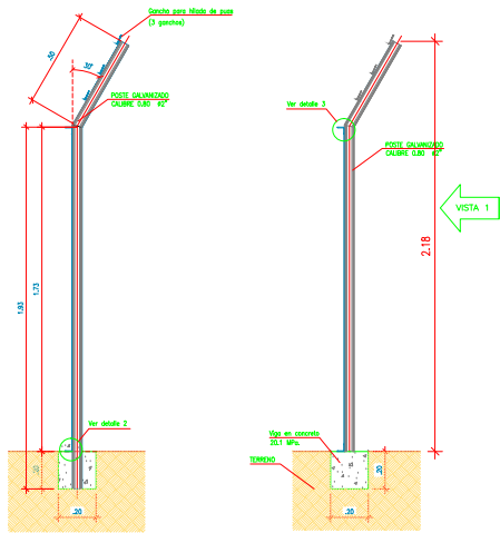
CORTE C'C 1:12.5
