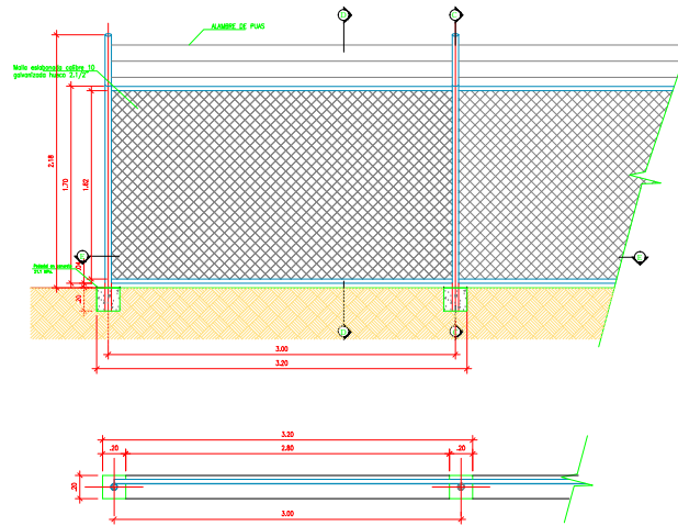
CORTE E'E CERRAMIENTO 1:20
