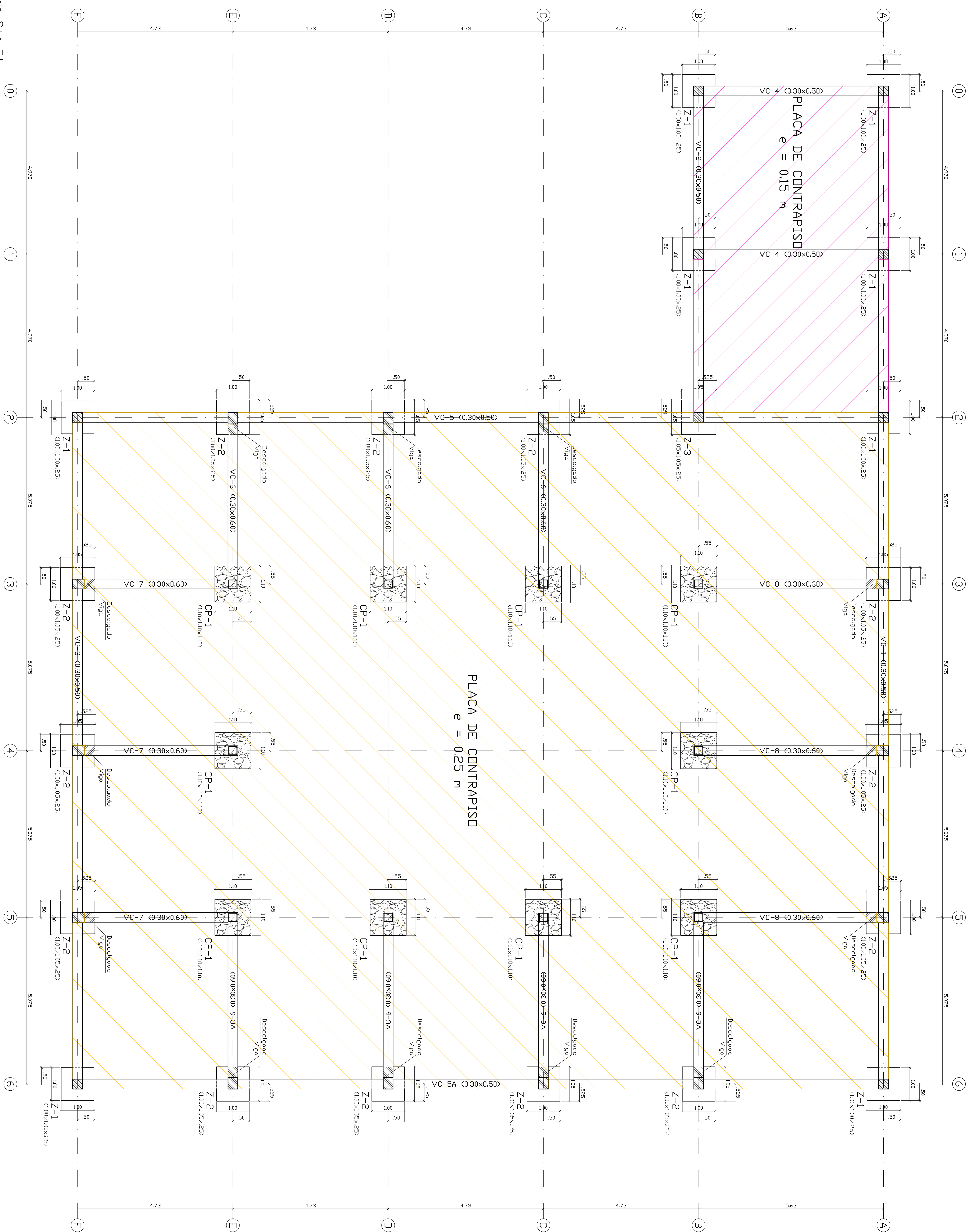
PLANTA CIMENTACION NIVEL Ne. -0.35
